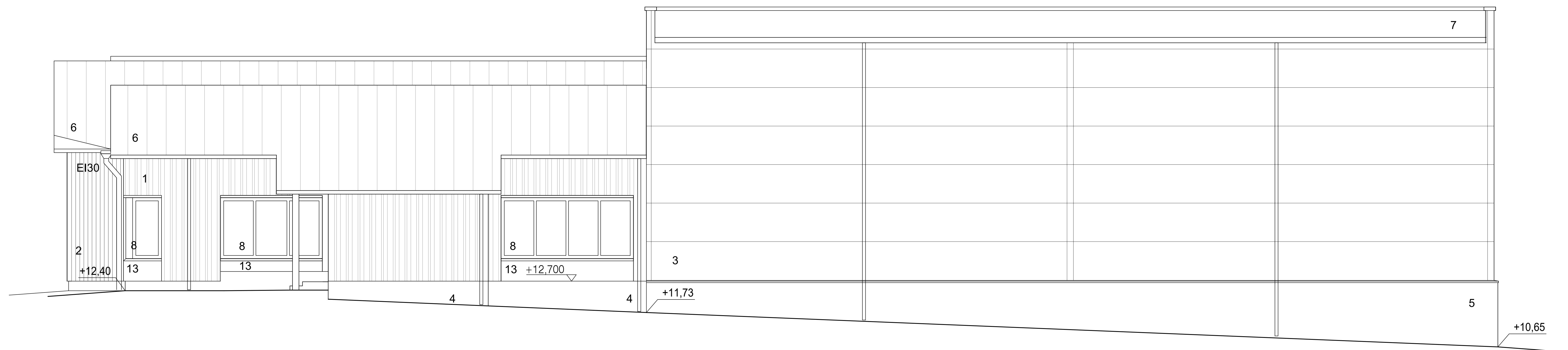
JULKISIVU LOUNAASEEN
