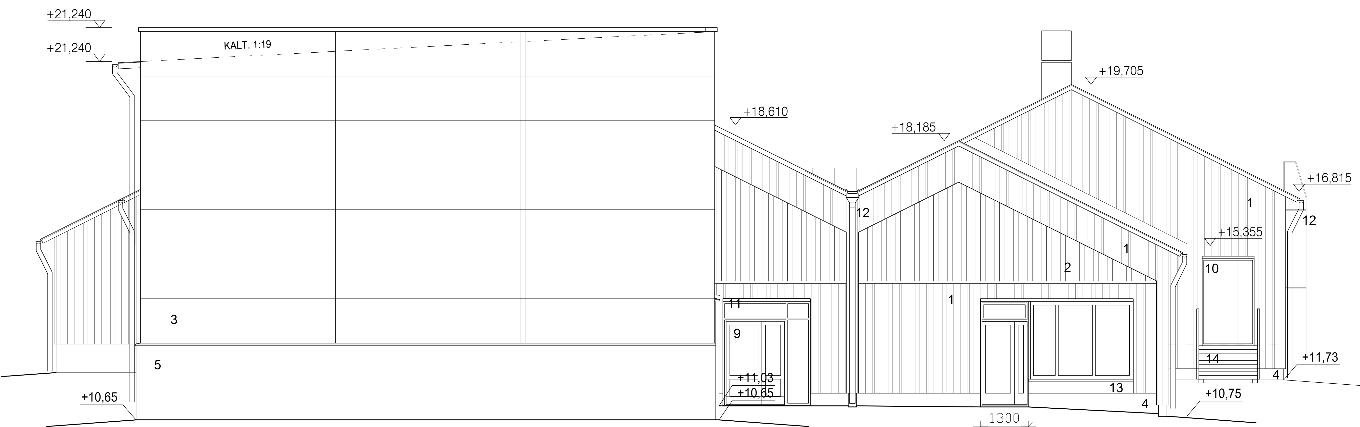
JULKISIVU KAAKKOON
