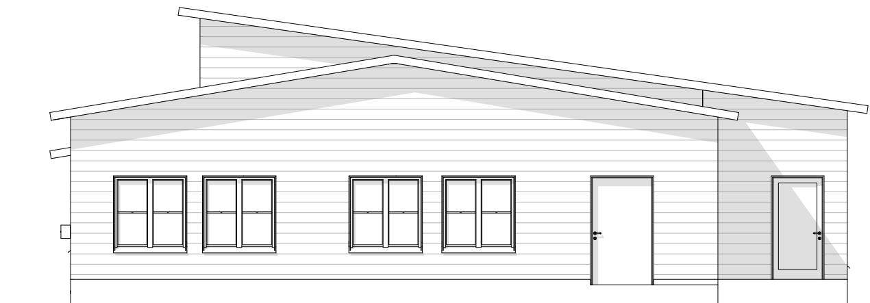
Julkisivu itään
