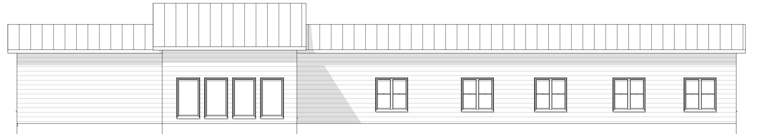
Julkisivu pohjoiseen
